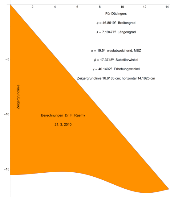
Abbildung 2 Zeigerdimensionen für die westabweichende Wand
