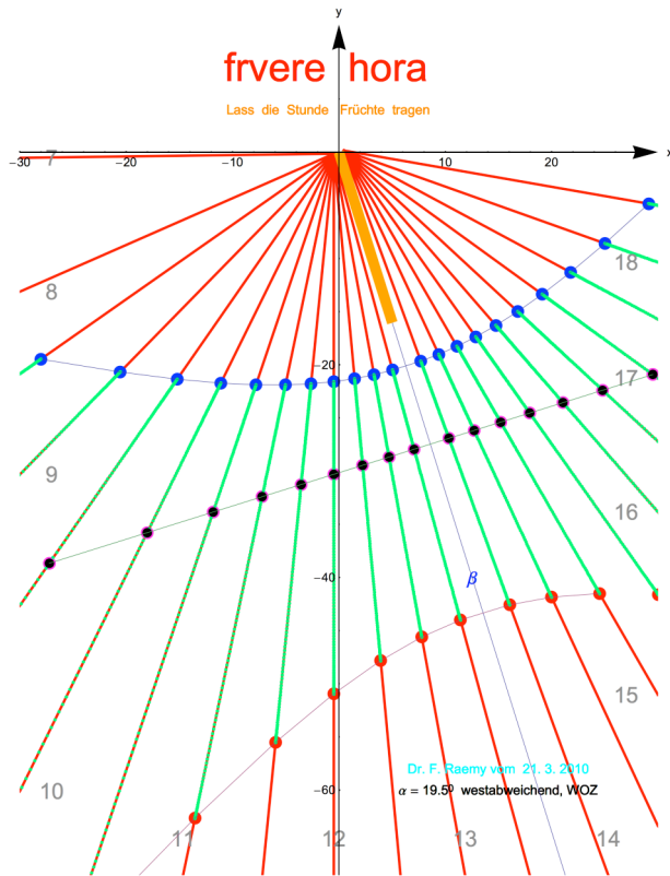
Abbildung 1 Zifferblatt an einer westabweichenden Wand
