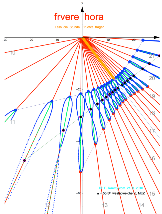
Abbildung 1 Zifferblatt an einer westabweichenden Wand
