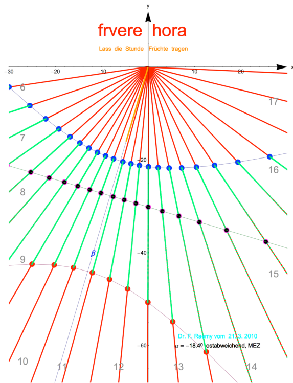
Abbildung 1 Zifferblatt an einer ostabweichenden Wand
