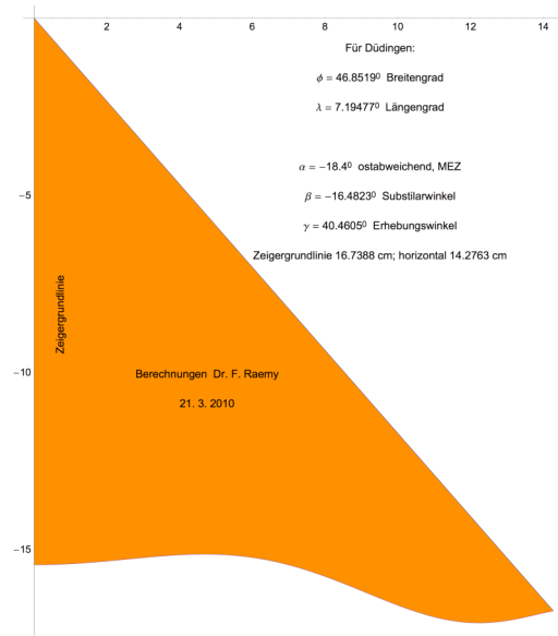
Abbildung 2 Zeigerdimensionen für die ostabweichende Wand
