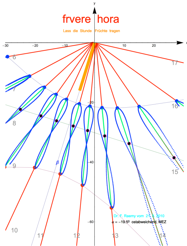
Abbildung 1 Zifferblatt an einer ostabweichenden Wand
