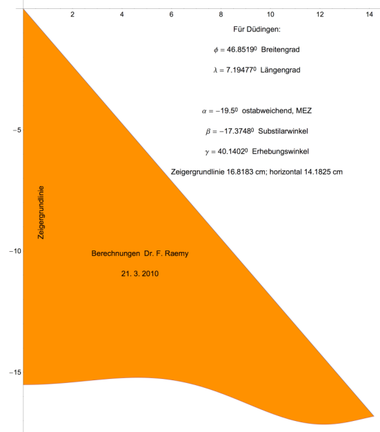
Abbildung 2 Zeigerdimensionen für die ostabweichende Wand
