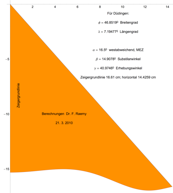
Abbildung 2 Zeigerdimensionen für die westabweichende Wand
