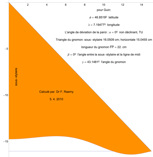
Figure 2 Les dimensions du gnomon
