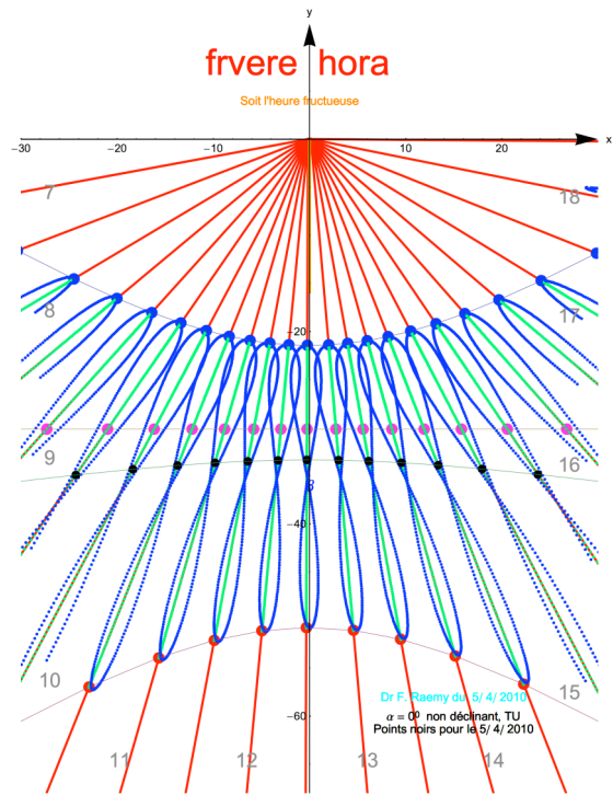
Figure 1 Le cadran solaire d'une paroi ouest – est
